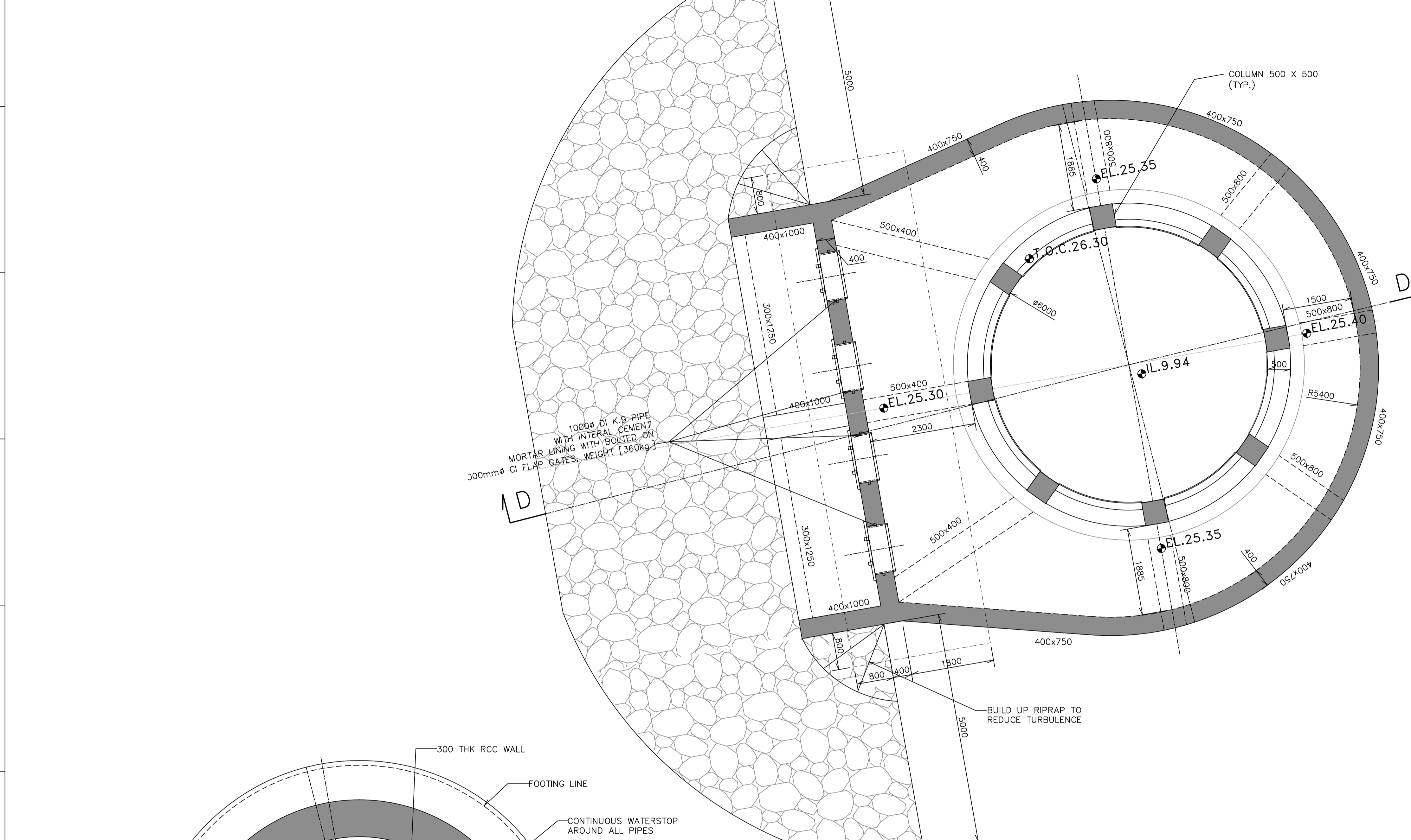
SECTIONAL PLAN B-B SCALE: 1:50
